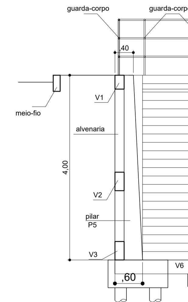
Corte A-A Escala 1:50
