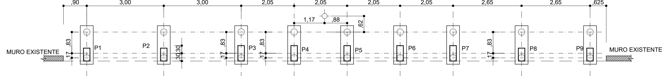
Locação de Pilares e Estacas Escala 1:75
