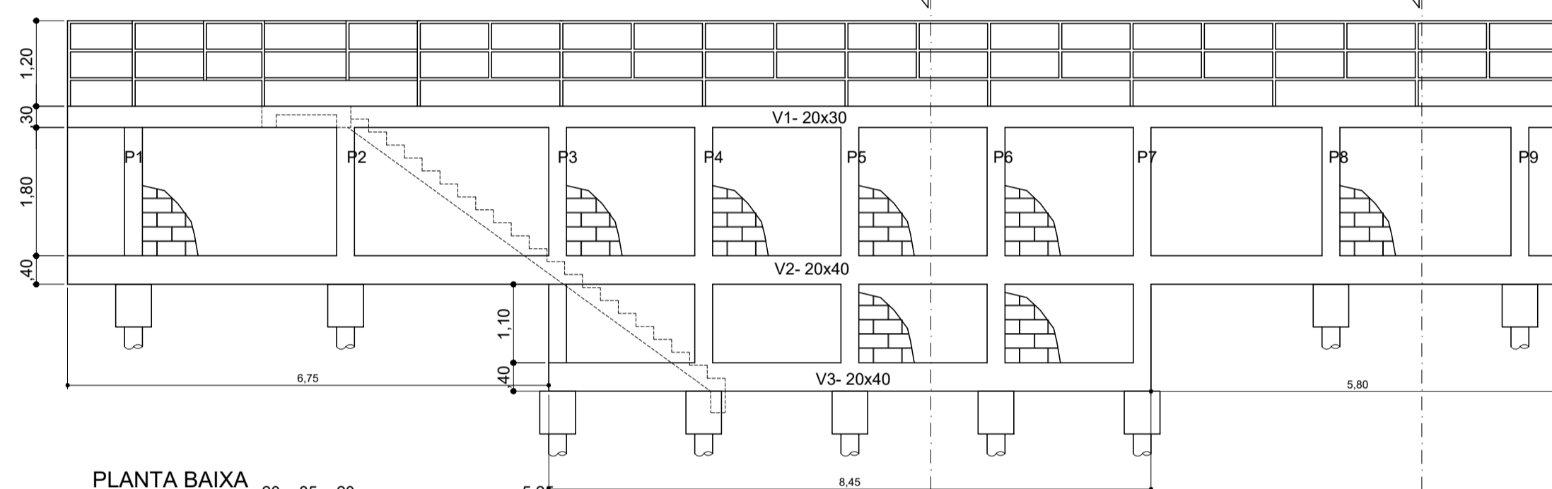
PLANTA BAIXA Escala 1:75
